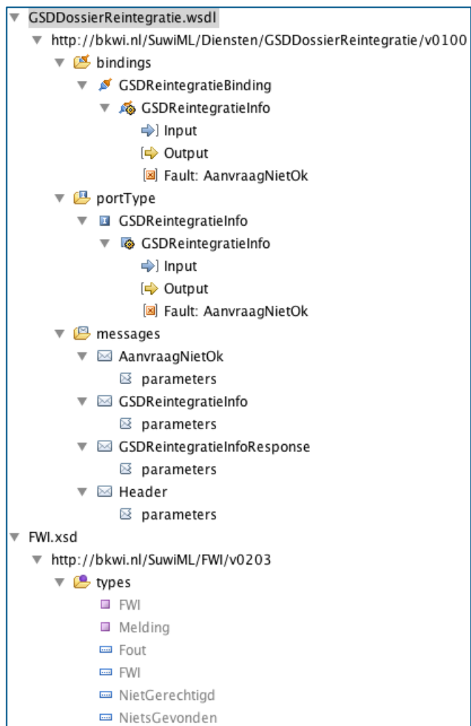
Afbeelding 17 Inhoud WSDL
