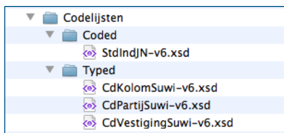
Afbeelding 12 Inhoud Codelijsten
